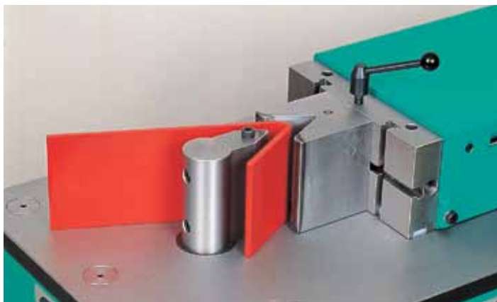
141 Prisma und Stempel 55° Vee-block and punch 55°
